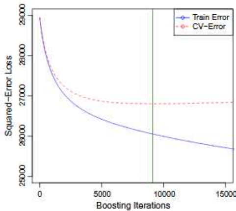
Gambar 4. Iterasi boosting
