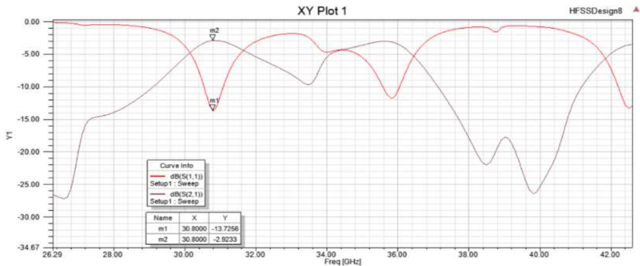
Gambar 22. Frekuensi Resonator Pada Grafik Parameter S_{11} dan S_{21} di 0,25 mm
