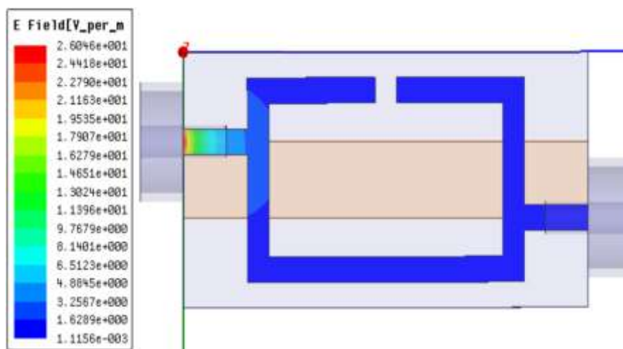
Gambar 8. Tampilan Magnitude Pada Bentuk Filter di 1 mm (Single Arm)
