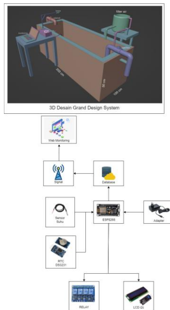
Gambar 7. Desain Sistem
