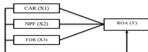
Gambar 1.1 Kerangka Pemikiran
