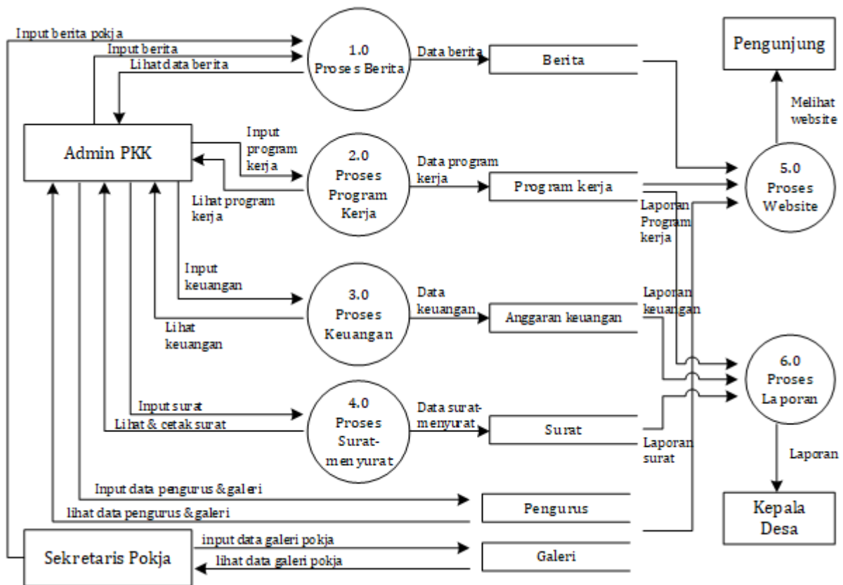
Gambar 5. Diagram Konteks
