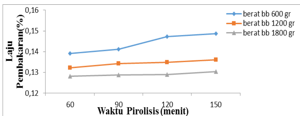
Gambar 6. Pengaruh berat bahan baku dan waktu terhadap laju pembakaran pada briket bioarang limbah padat nilam.
