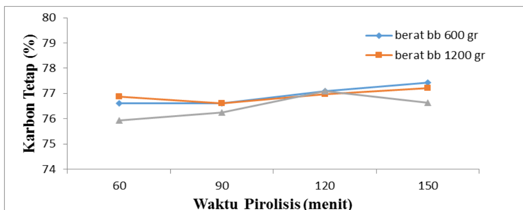
Gambar 5. Pengaruh berat bahan baku dan waktu terhadap kadar karbon tetap pada briket bioarang limbah padat nilam.
