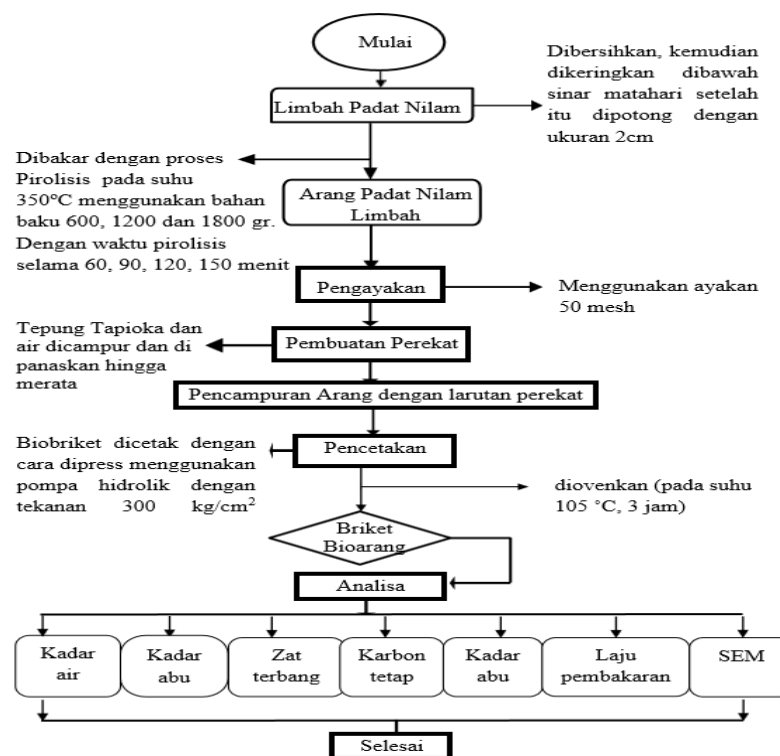
Gambar 1 Diagram Pembuatan Briket Bioarang Limbah Padat Nilam
