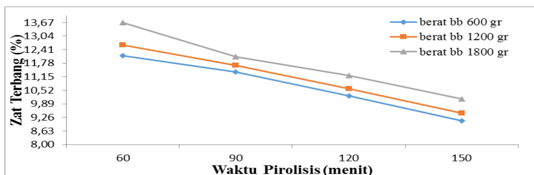
Gambar 4. Pengaruh berat bahan baku waktu terhadap zat terbang pada briket bioarang limbah padat nilam
