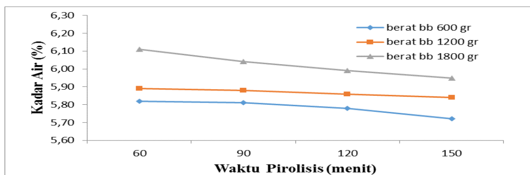
Gambar 2. Pengaruh berat bahan baku dan waktu terhadap kadar air pada briket bioarang limbah padat nilam
