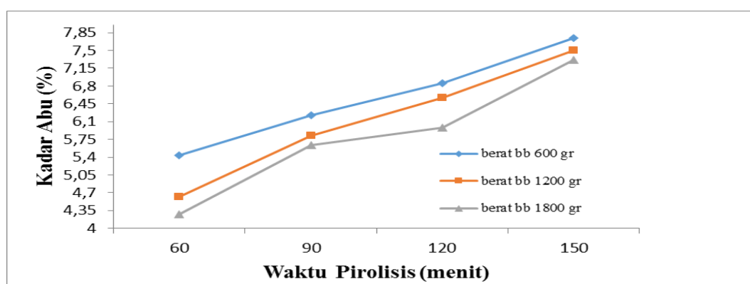
Gambar 3. Pengaruh berat bahan baku waktu terhadap kadar abu pada briket bioarang limbah padat nilam
