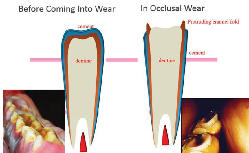
Gambar 8. Diagram pemanjangan gigi lebih lanjut. Dengan pemanjangan lebih lanjut, gigi sekarang menjadi hypsodont. Saat erupsi, mahkota klinis sepenuhnya ditutupi email dengan sementum di atasnya, yaitu permukaan hypsodont primer (gambar permukaan primer gigi pipi mandibula neonatal di sebelah kiri). Begitu gigi mulai aus, sementum dan email pada permukaan oklusal cepat terkikis sehingga memperlihatkan tonjolan email pada permukaan oklusal hypsodont permanen (gambar gigi pipi mandibula dewasa di sebelah kanan). lipatan email menonjol di antara sementum dan dentin yang lebih lunak, dalam mekanisme penajaman sendiri (Scott Pirie dalam MacFadden BJ, 2014).
