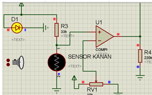
Gambar 6. Rangkaian Sensor
