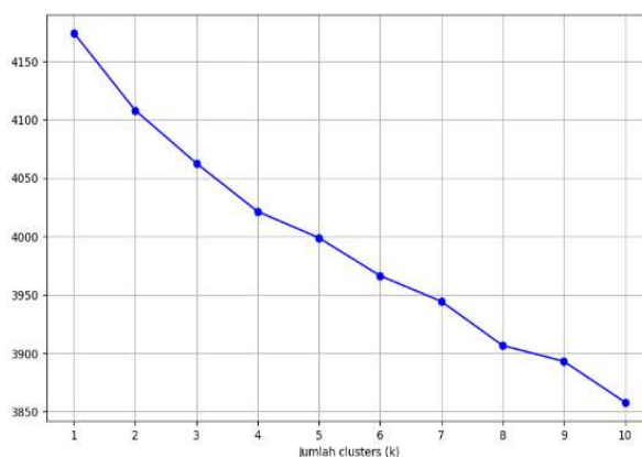
Gambar 4. Hasil Grafik Elbow
