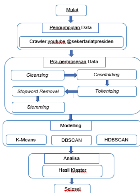
Gambar 1. Tahapan Metode Penelitian
