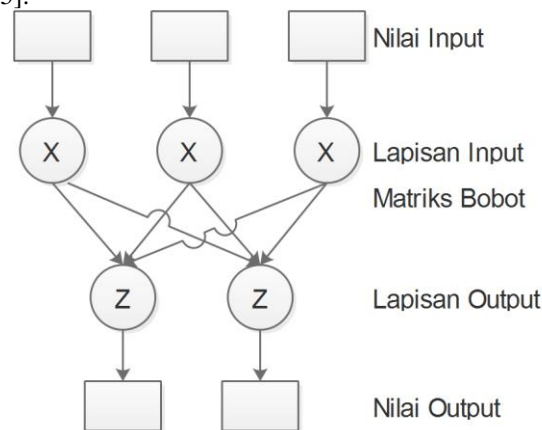
Gambar 1 Layer JST
