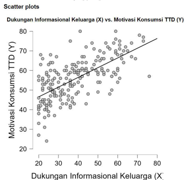
Gambar 1. Scatter Plots Hubungan Dukungan Informasional Keluarga dengan Motivasi Konsumsi TTD
