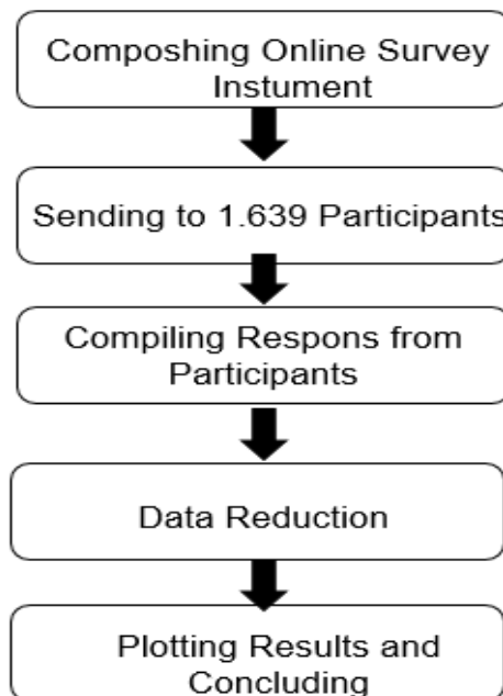
Gambar 1. Metodologi Penelitian
