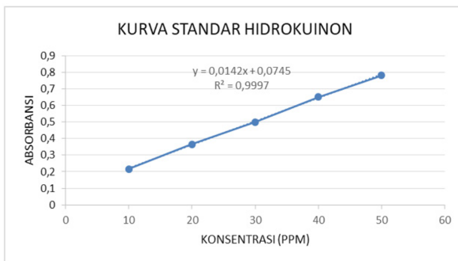
Gambar 1 Kurva Baku Hidrokuinon Sumber: Data Diolah
