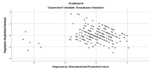
Gambar 2. Uji Heteroskedastisitas
