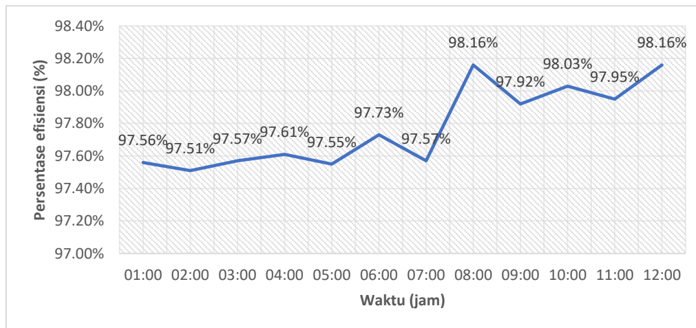
Gambar 1. Grafik Efisiensi Transformator GT Unit 1
