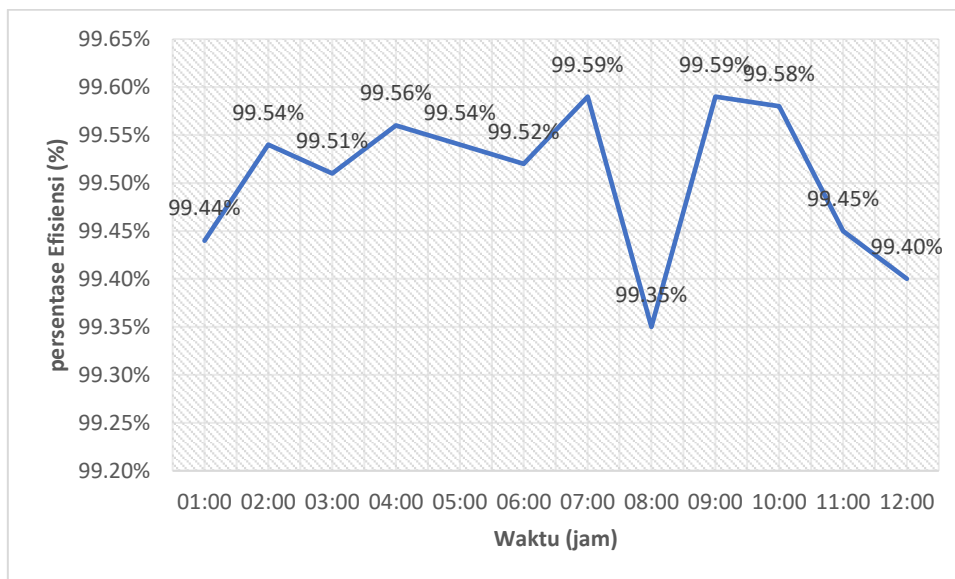
Gambar 2. Grafik Efisiensi Transformator GT Unit
