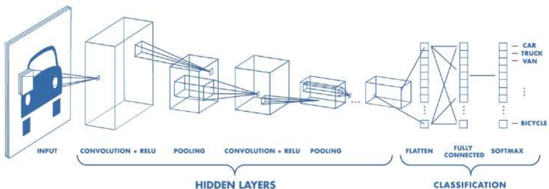
Gambar 1. CNN
