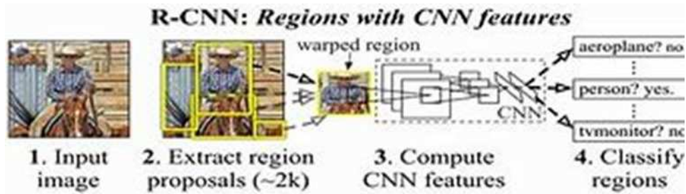
Gambar 2. R-CNN
