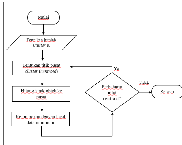
Gambar 2.3 Alur Algoritma K-Means
