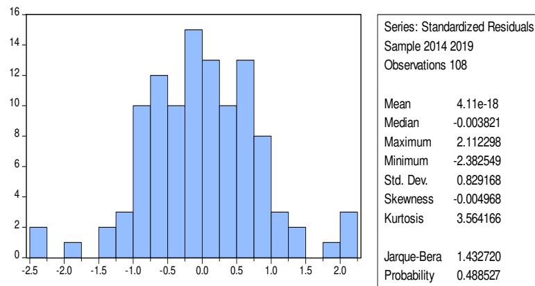
Gambar 2. Uji Normalitas
