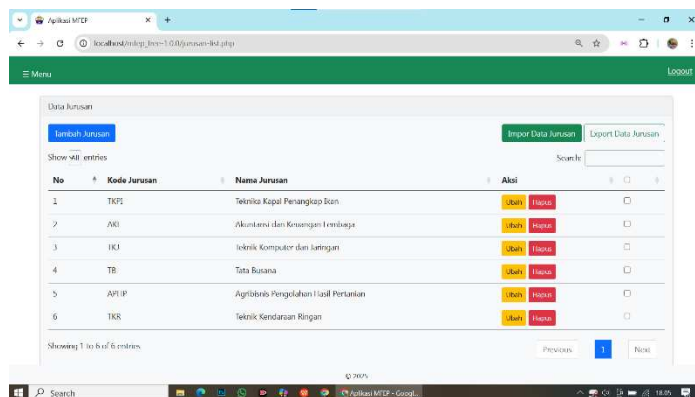
Gambar 8. Jurusan
