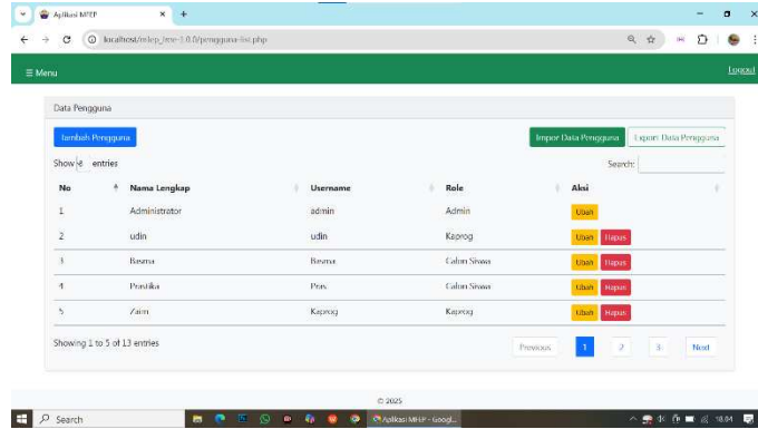
Gambar 7. Pengguna
