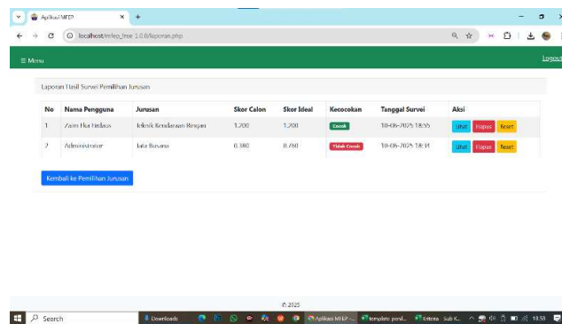
Gambar 11. Laporan
