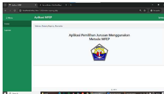
Gambar 15. Dashboard Kaprog
