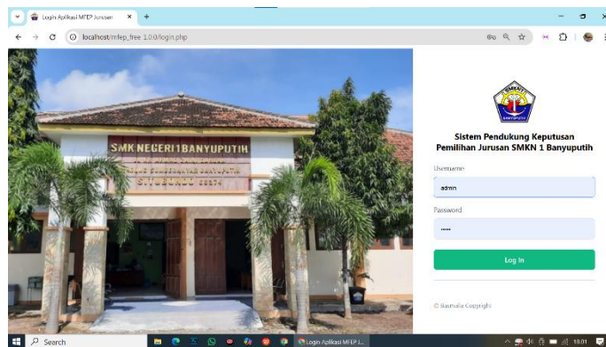
Gambar 5. Halaman Login
