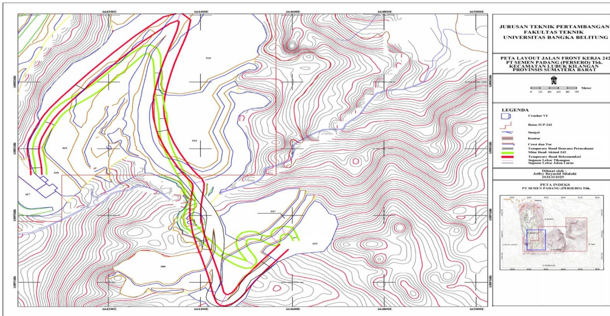
Lampiran 1. Design perbaikan geometri jalan
