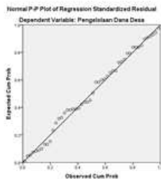
Gambar 2. Grafik Histogram
