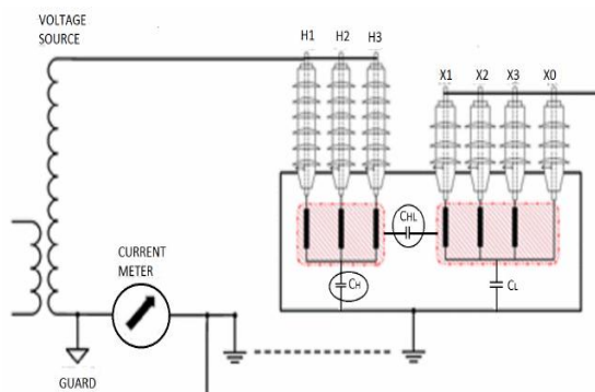
Gambar 4. Hubungan rangkaian pengujian tan \Delta test
