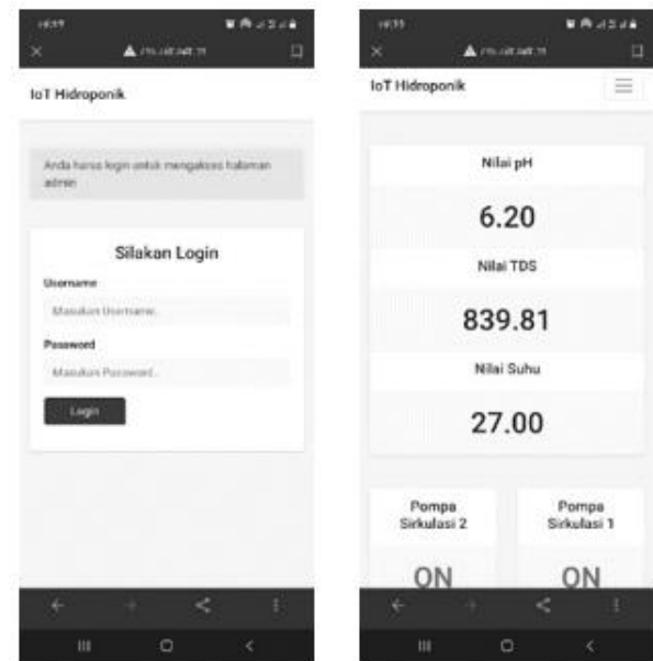
Gambar 7. Tampilan Aplikasi Web
