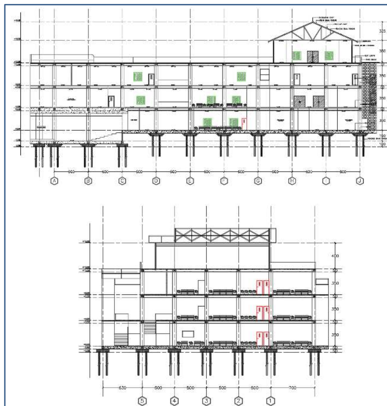
Gambar 10 : Potongan Memanjang & Melintang Sumber : Analisa Penulis
