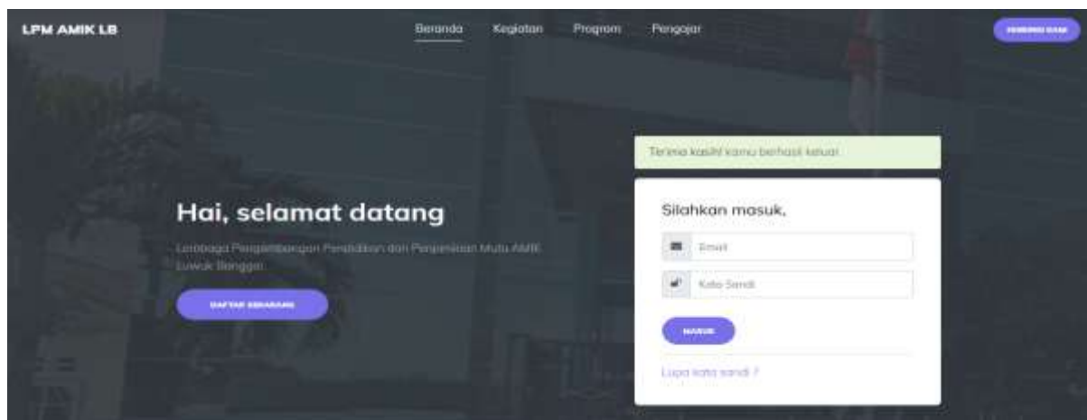
Gambar 4. Halaman Login .
