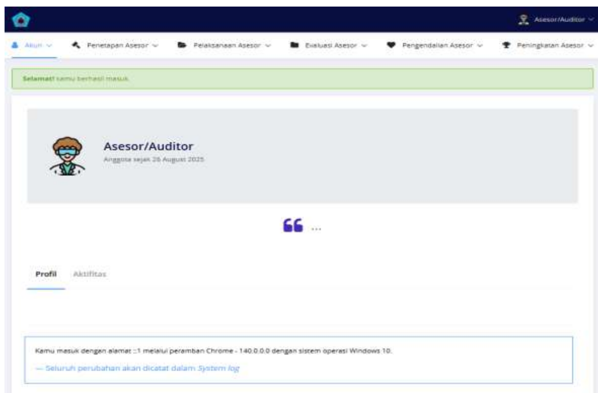
Gambar 7. Halaman Asesor.
