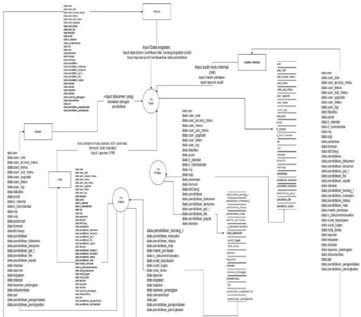
Gambar 3. DFD.
