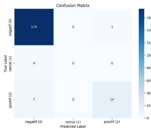
Gambar 7. SVM
