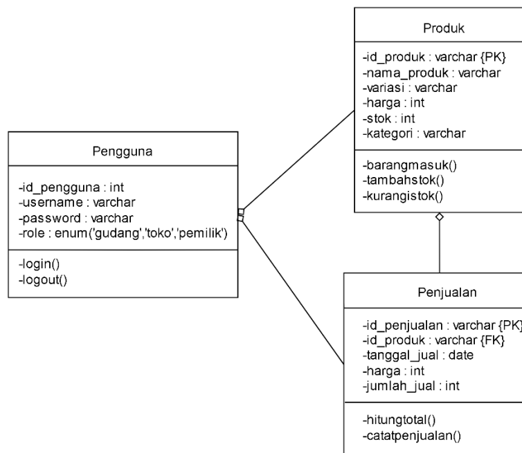
Gambar 2. Class Diagram Sistem Informasi Penjualan
