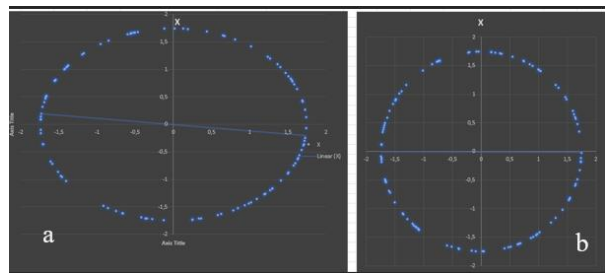
Gambar 5. Hasil Offset pengukuran Kompas Digital a. sebelum kompensasi dan b. setelah kompensasi
