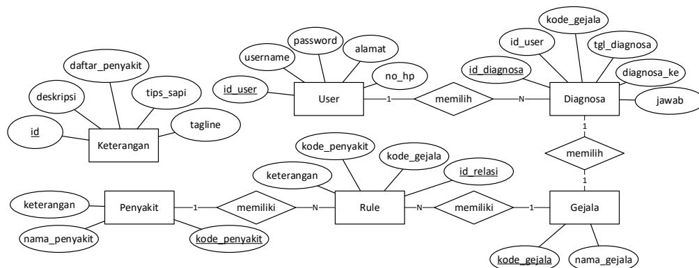
Gambar 3. ERD
