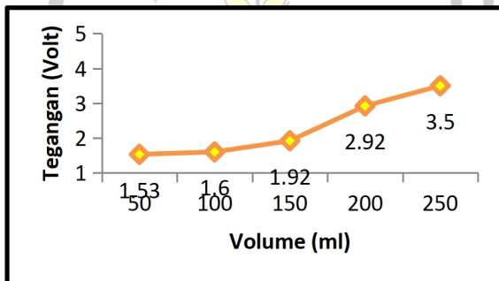
Gambar 2. Grafik Hubungan Variasi Penambahan Volume Terhadap Nilai Tegangan Listrik Larutan Kulit Nenas
