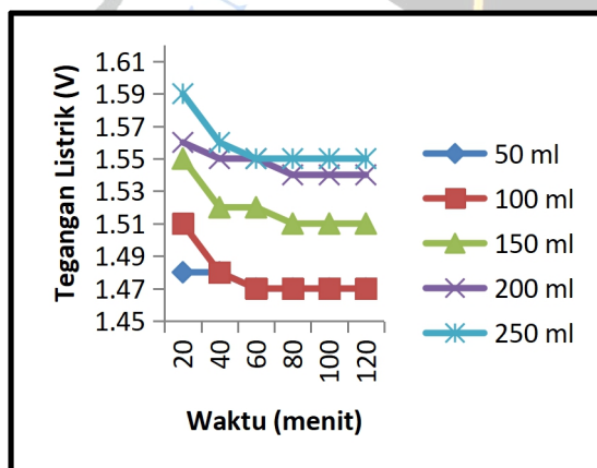
Gambar 4. Grafik Penurunan Tegangan dari Larutan Kulit Nenas Selama 2 Jam
