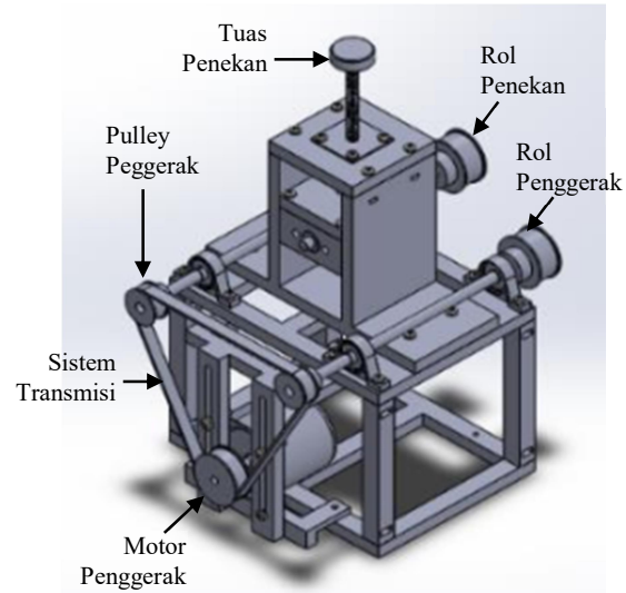
Gambar 5. Prototipe Mesin Rol Pelat
