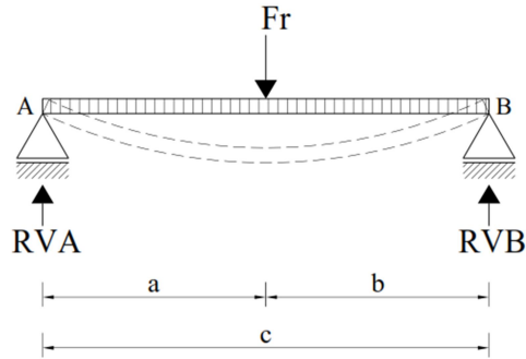
Gambar 7. Analisa Konsep keseimbangan Benda Uji.
