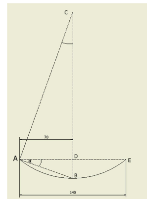
Gambar 12. Radius lengkung pelat.
