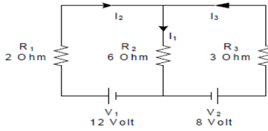
Gambar 2. Rangkaian listrik
