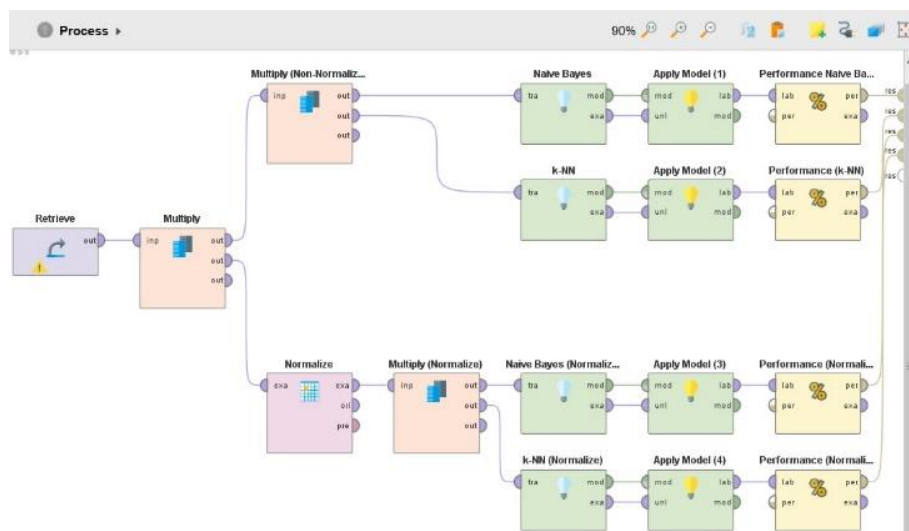
Gambar 3 Proses Data Penyakit Jantung
