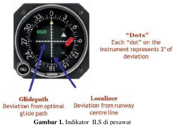
Gambar 1. Indikator ILS di pesawat
