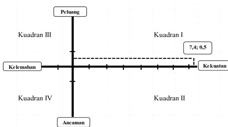
Gambar 1 Matrik posisi strategi peningkatan respons peternakan domba
