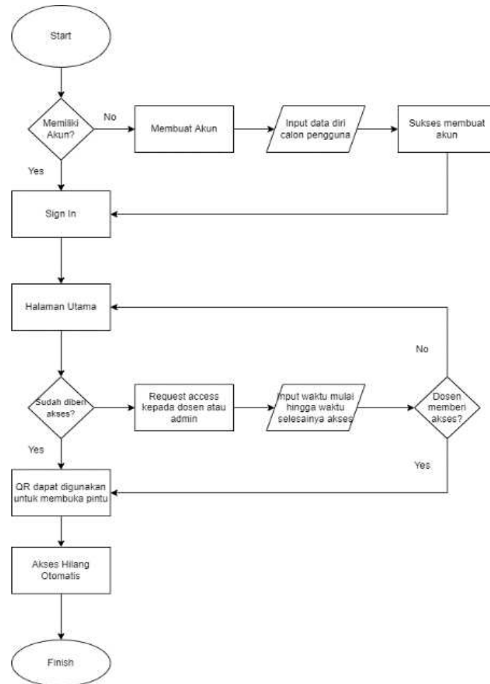
Gambar 1. Bagan Alur Cara Kerja Aplikasi Secure Lab
