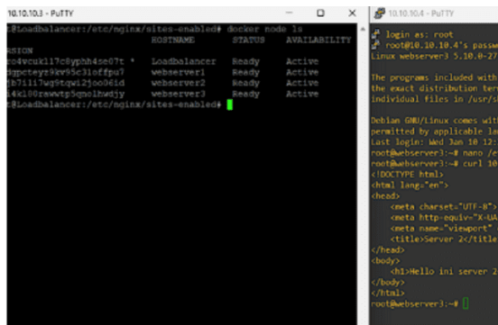
Gambar 11. sistem berhasil mengalihkan request dari IP selain 10.10.10.11 ke server 2
