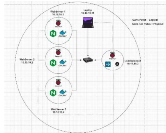
Gambar 2. Desain Perancangan Sistem
