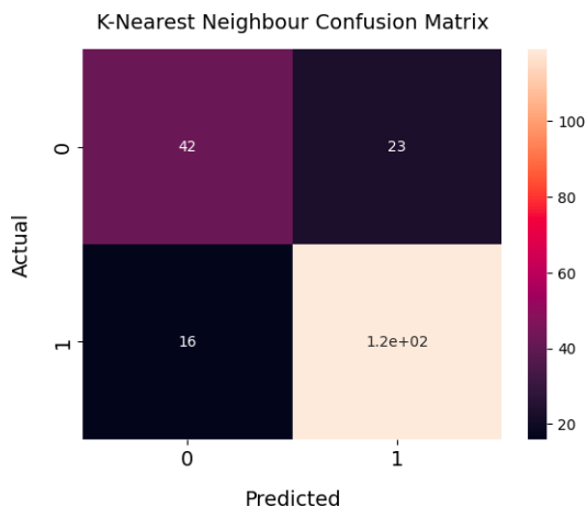
Gambar 3. Hasil Algoritma KNN
