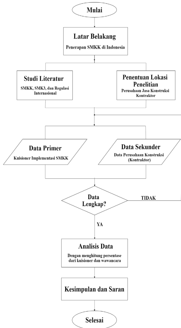
Gambar 1. Tahapan Penelitian
