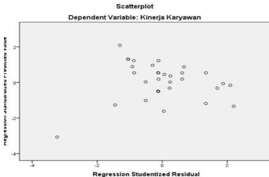
Gambar 6. Uji Heterodastisitas dari SPSS Sumber: Hasil Pengolahan data SPSS Ver 21
