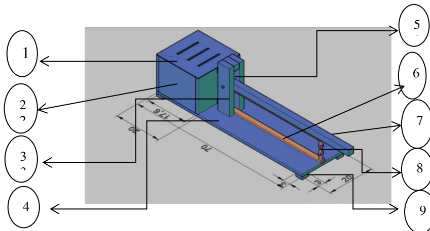
Gambar 15 Rancangan Keseluruhan Alat Las Titik ( SpotWelding )
