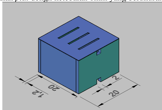
Gambar 10 Rancangan kotak tempat trafo
