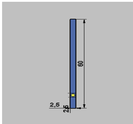
Gambar 12 Rancangan stang las
