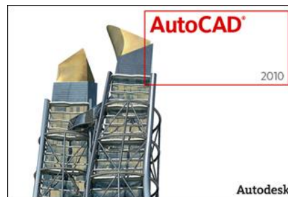
Gambar 7 AutoCAD 2010
