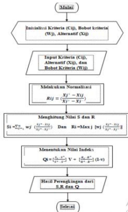
Gambar 3.2 Flowchart Metode VIKOR.
