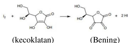
Gambar 3. Reaksi asam askorbat dengan Iodium
