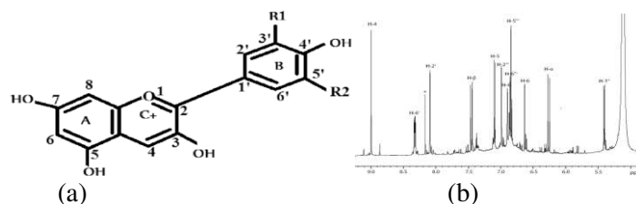
Gambar 5. (a) Struktur Antosianin (b) Karakterisasi ^1H NMR Antosianin
