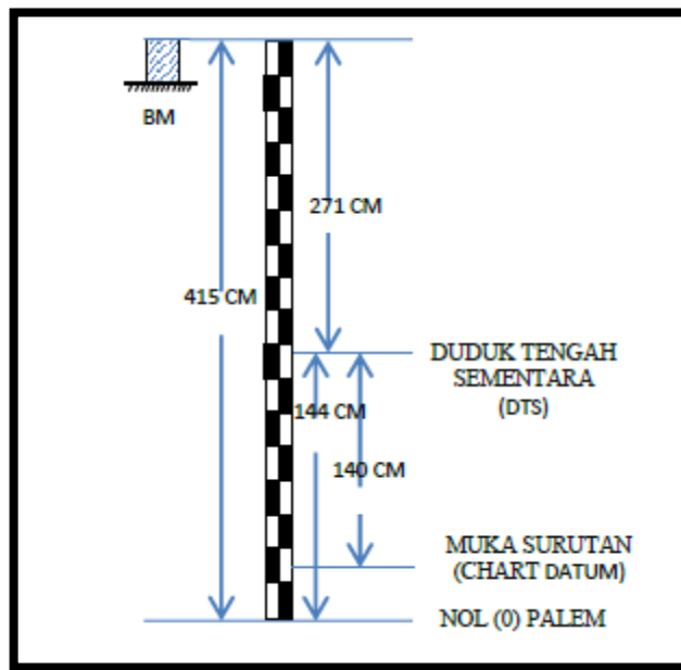
Gambar 3. Sketsa kedudukan BM terhadap Nol Palem
