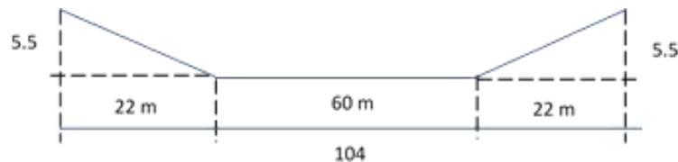
Gambar 6. Desain penampang keruk
