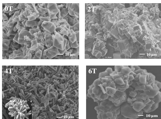
Gbr 2. Gambar SEM dari Zn-oxac-ATaz or [\text{Zn}_2(\text{C}_2\text{O}_4)(\text{C}_2\text{N}_4\text{H}_2)_2] \cdot (\text{H}_2\text{O})_{0.5} yang dibuat dalam berbagai kekuatan medan magnet; 0T, 2T, 4T and 6T
