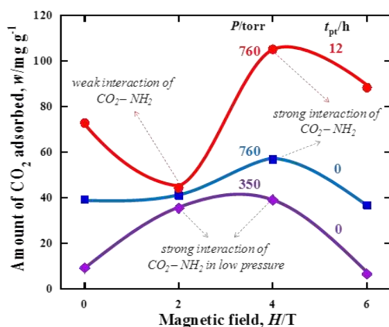
Gbr 6. Adsorpsi \text{CO}_2 dari Zn-oxac-ATaz yang dibuat dalam berbagai kekuatan medan magnet, tanpa perlakuan awal dan dengan perlakuan awal selama 12h
