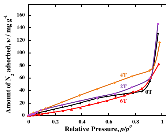
Gbr 3. Adsorpsi \text{N}_2 adsorption dari [\text{Zn}_2(\text{C}_2\text{O}_4)(\text{C}_2\text{N}_4\text{H}_2)_2] \cdot (\text{H}_2\text{O})_{0.5} atau Zn-oxac-ATaz pada 77K setelah pretreatment pada 110 °C selama 12h and disintesis pada berbagai kekuatan medan magnet; 0T, 2T, 4T and 6T
