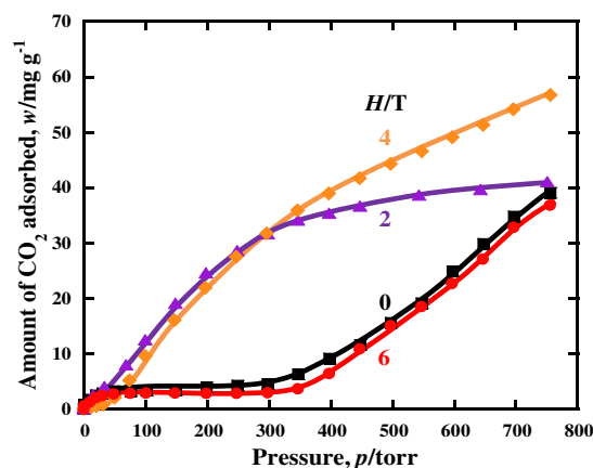
Gbr 4. Adsorpsi \text{CO}_2 pada Zn-oxac-ATaz atau [\text{Zn}_2(\text{C}_2\text{O}_4)(\text{C}_2\text{N}_4\text{H}_2)_2] \cdot (\text{H}_2\text{O})_{0.5} pada 333K tanpa pretreatment, dibuat dalam berbagai kekuatan medan magnet; 0T, 2T, 4T and 6T.
