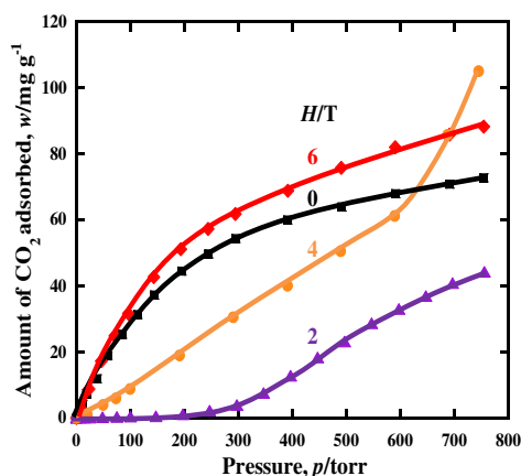
Gbr 5. Adsorpsi gas \text{CO}_2 pada 30^\circ\text{C} [\text{Zn}_2(\text{C}_2\text{O}_4)(\text{C}_2\text{N}_4\text{H}_2)_2] \cdot (\text{H}_2\text{O})_{0.5} atau Zn-oxac-ATaz pada 77K setelah perlakuan awal pada 110^\circ\text{C} selama 12h and dibuat dalam berbagai kekuatan medan magnet; OT, 2T, 4T and 6T
