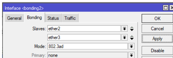
Sumber : Penelitian (2025) Gambar 6. Konfigurasi Bonding CRS lantai 3
