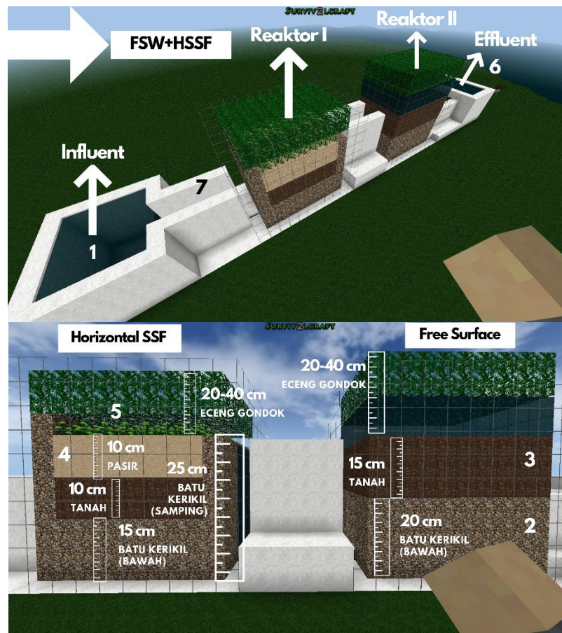
Gambar 1 Rangkaian Alat
