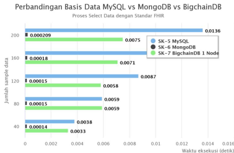
Gambar 10 Grafik perbandingan select data dengan standar FHIR.
