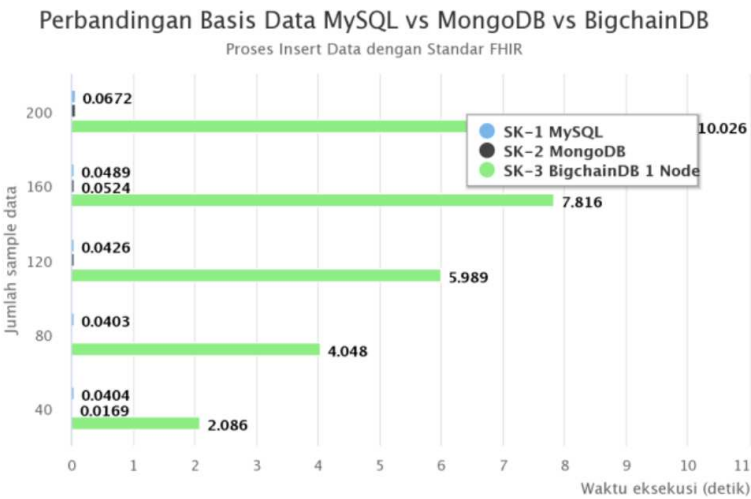
Gambar 9 Grafik perbandingan insert data dengan standar FHIR.
