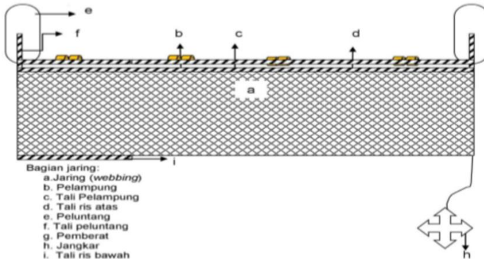
Gambar lengkap Gill net Monofilament setelah dirangkai lengkap
