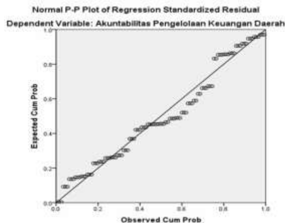
Gambar 2 Uji Normalitas
